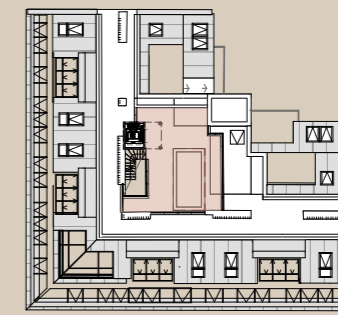
DACHDRAUFSICHT
