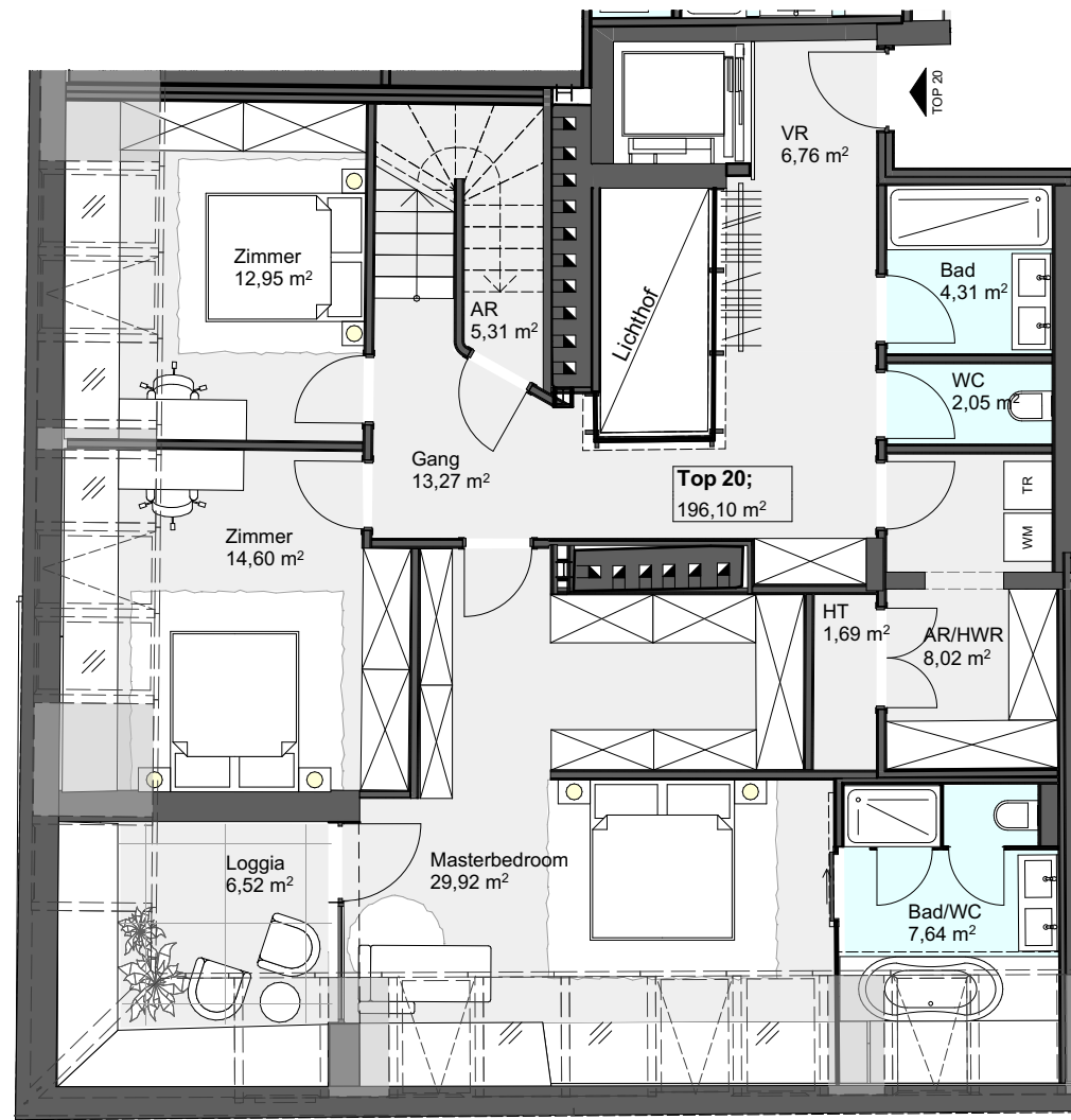
1. DACHGESCHOSS
