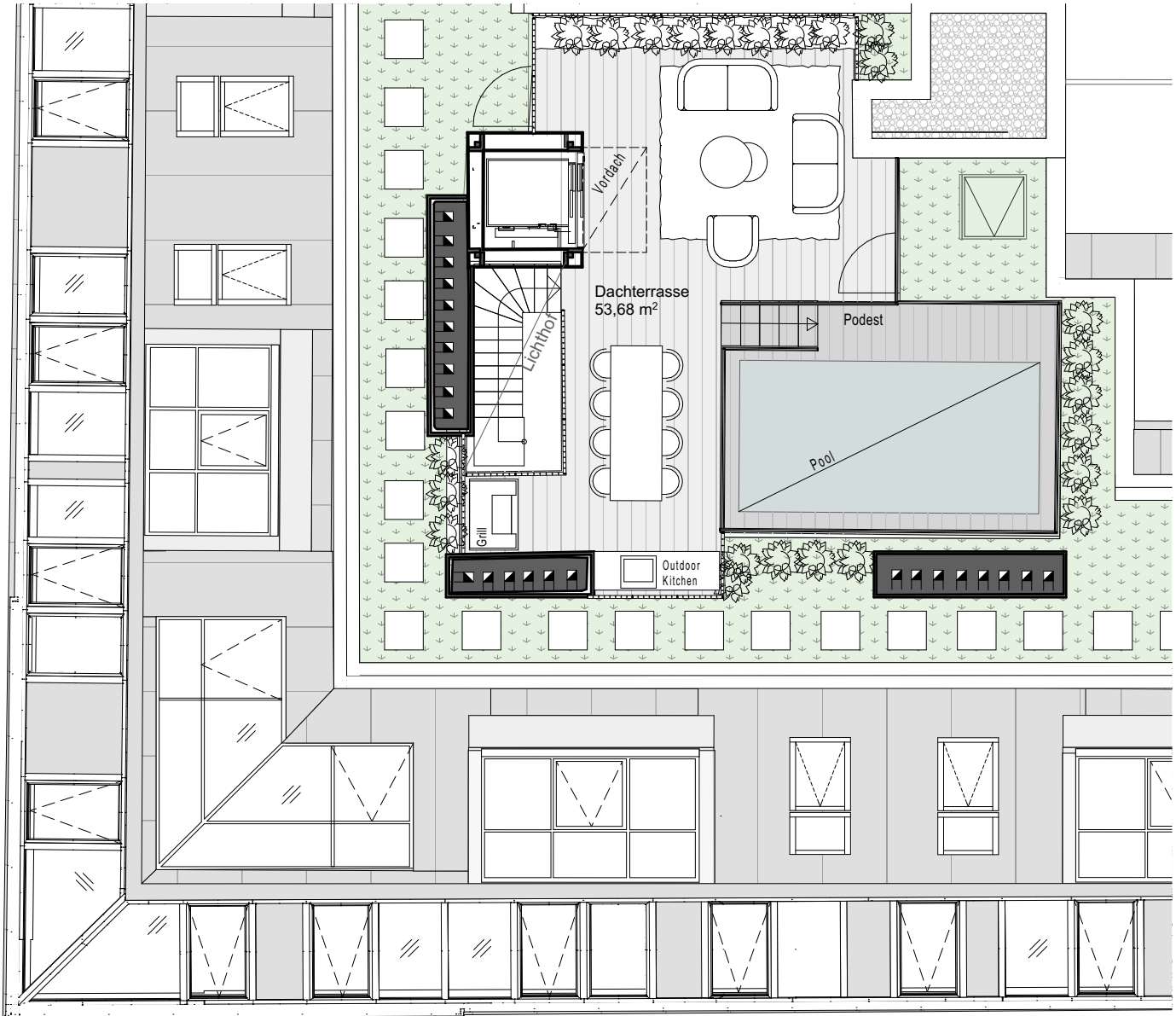
DACHDRAUFSICHT
