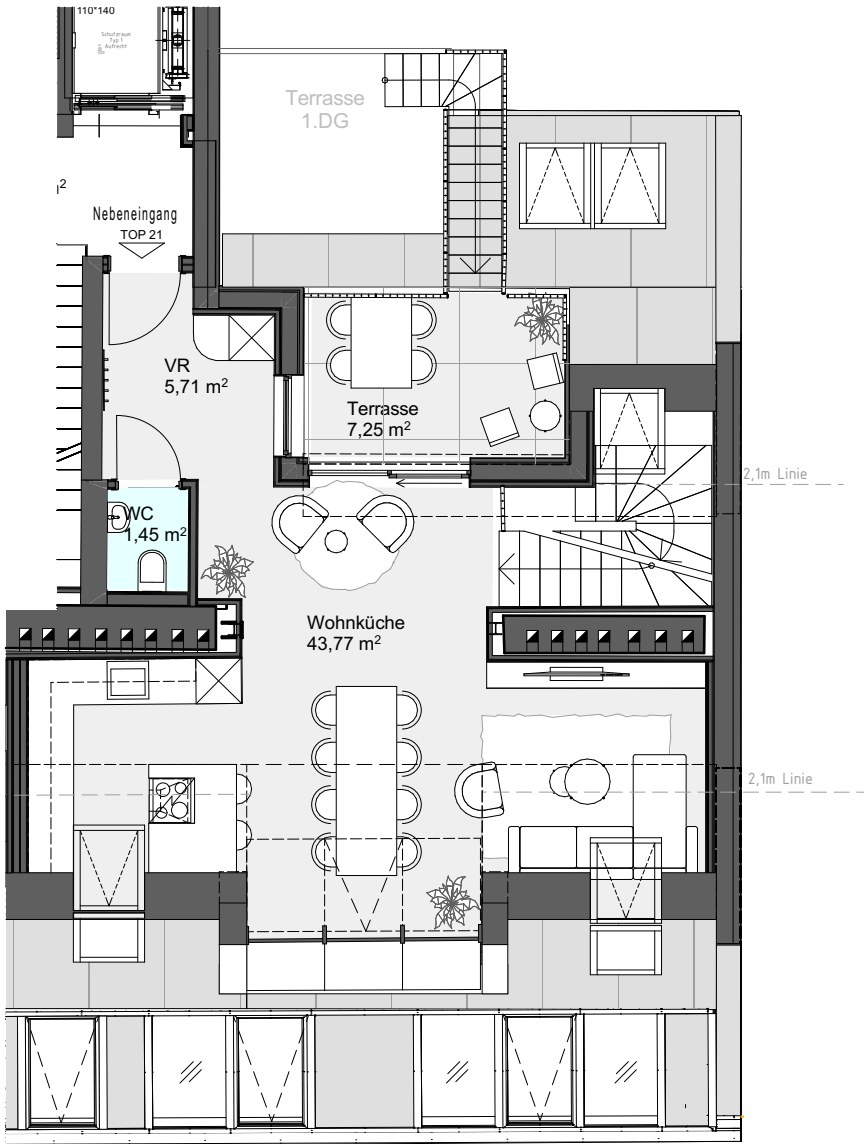
2. DACHGESCHOSS
